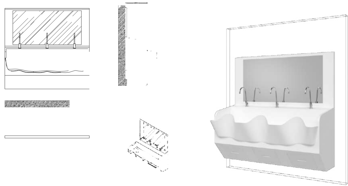
Trojité závěsné umyvadlo RLM-G086 Rozměry: Š 1800 mm × V 1970 mm × H 775 mm
