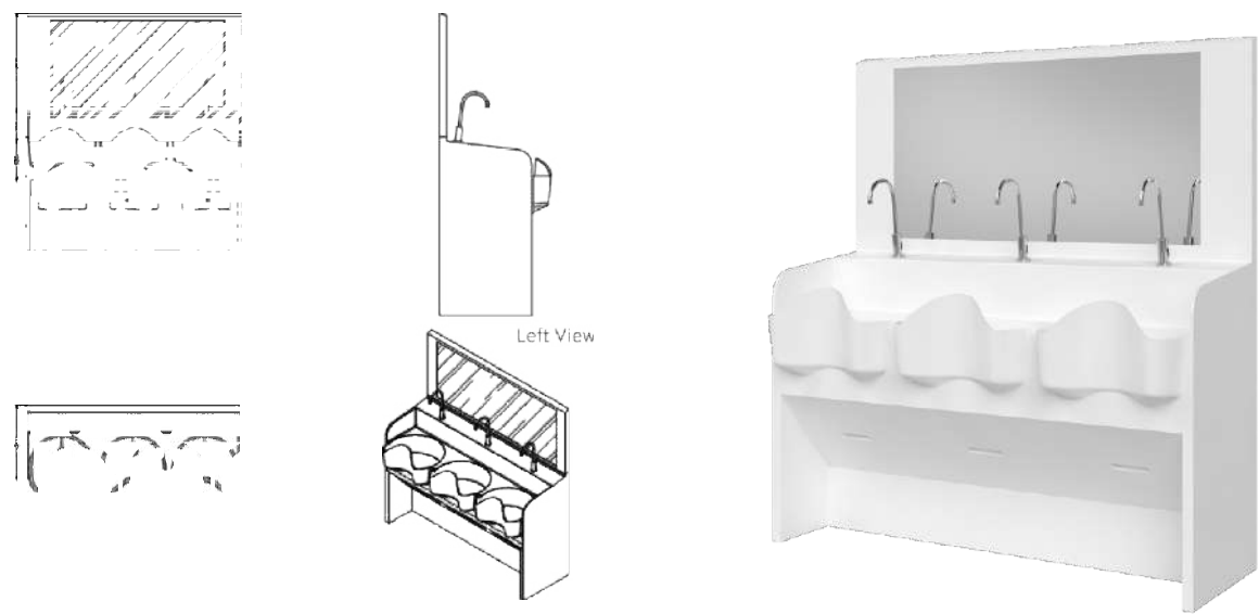
Podlahové trojité umyvadlo RLM-G071 Rozměry: Š 800 mm × V 1970 mm × H 722 mm
