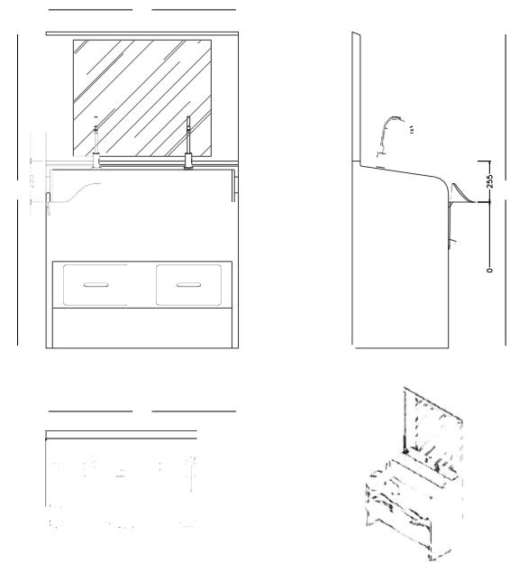
Dvojité umyvadlo stojící na podlaze RLM-G049 Rozměry: Š 1200 mm × V 1970 mm × H 775 mm
