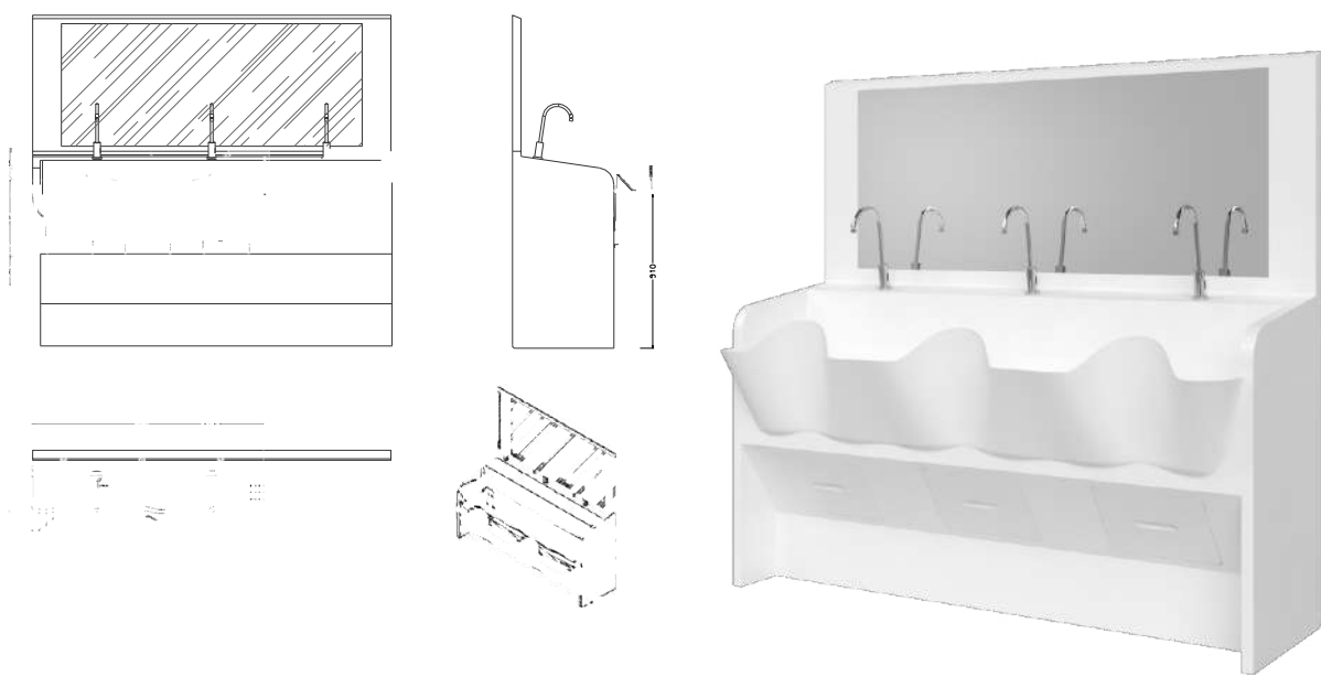
Trojité umyvadlo stojící na podlaze RLM-G005 Rozměry: Š 2120 mm × V 1970 mm × H 775 mm
