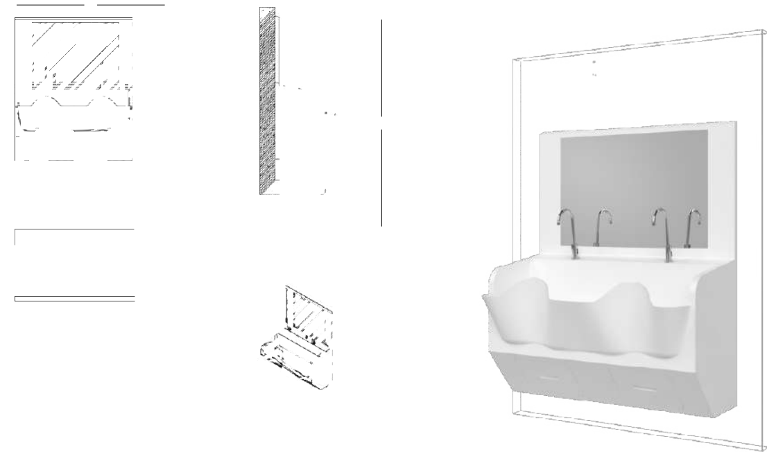
Dvojité závěsné umyvadlo RLM-G048 Rozměry: H 1420 mm × V 1970 mm × Š 775 mm
