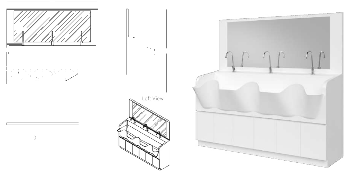
Trojité umyvadlo s umyvadlovou skříňkou RLM-G001 Rozměry: Š 2120 mm × V 1970 mm × H 770 mm
