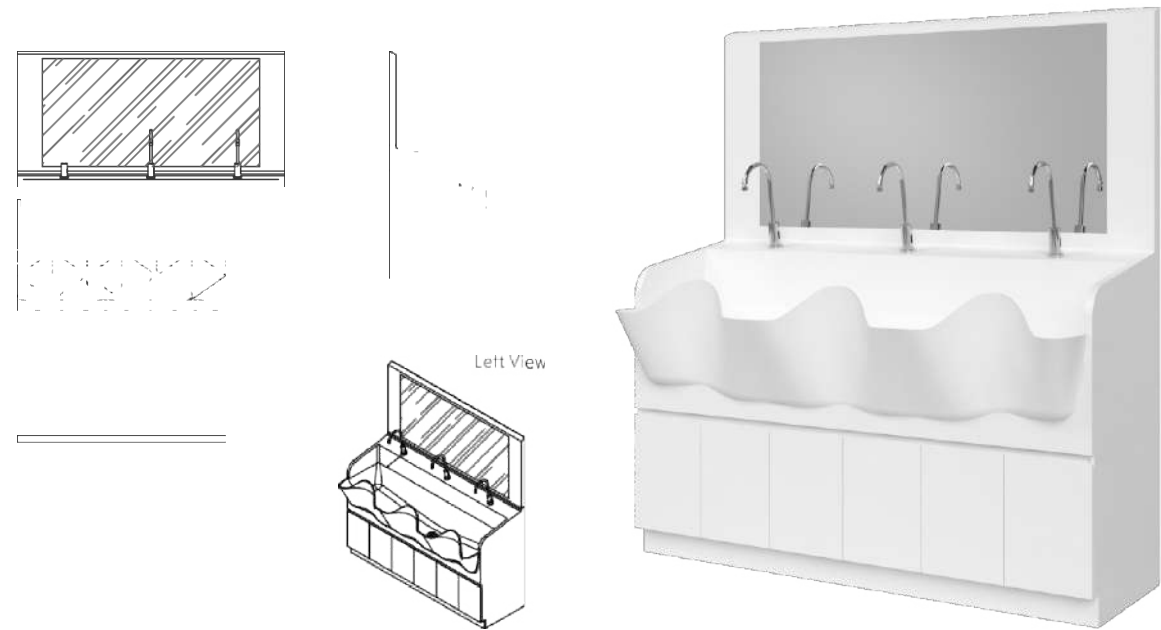
Trojité umyvadlo s umyvadlovou skříňkou RLM-G059 Rozměry: Š 1800 mm × V 1970 mm × H 775 mm
