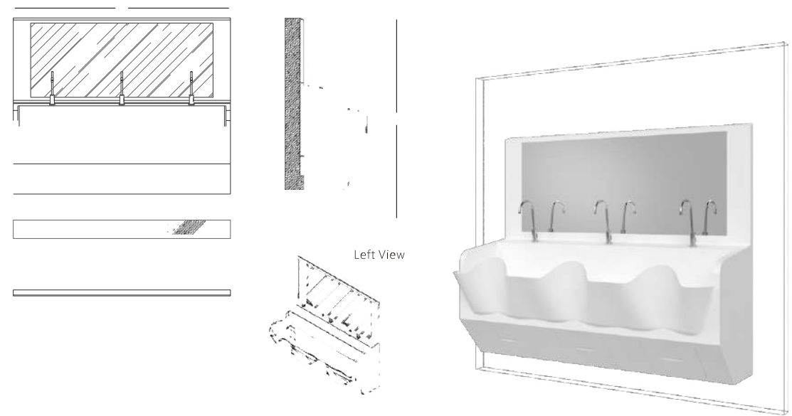
Trojité závěsné umyvadlo RLM-G057 Rozměry: Š 2120 mm × V 1970 mm × H 775 mm
