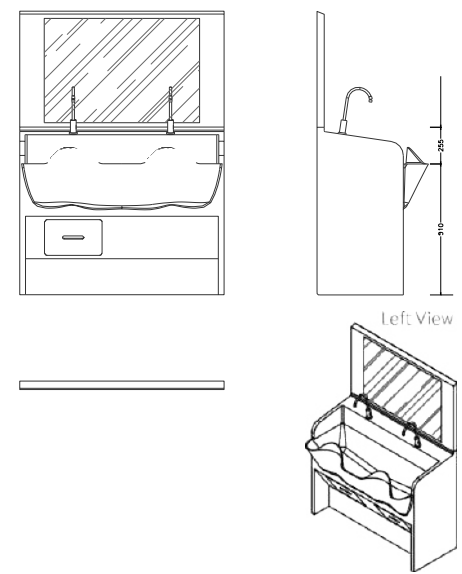
Dvojité umyvadlo stojící na podlaze RLM-G021 Rozměry: Š 1420 mm × V 1970 mm × H 775 mm
