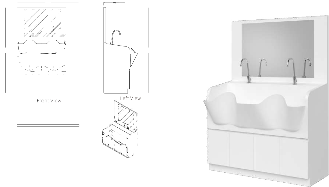
Dvojité umyvadlo s umyvadlovou skříňkou RLM-G017 Rozměry: Š 1420 mm × V 1970 mm × H 775 mm
