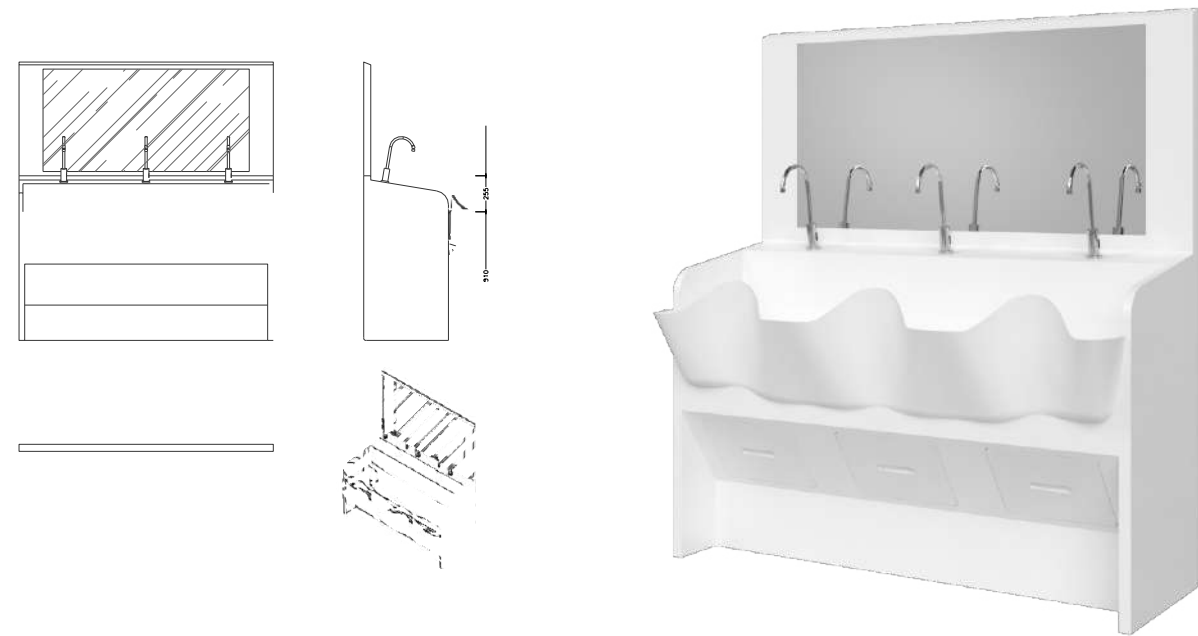
Trojité umyvadlo stojící na podlaze RLM-G058 Rozměry: Š 1800 mm × V 1970 mm × H 775 mm
